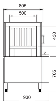
VISTA LATERAL
