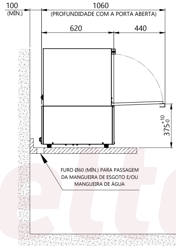
VISTA LATERAL
