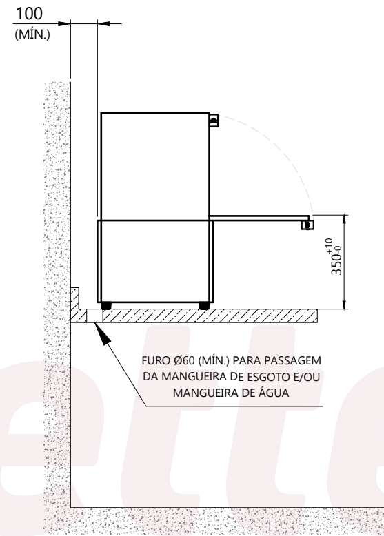
VISTA LATERAL
