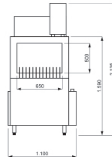
VISTA LATERAL
